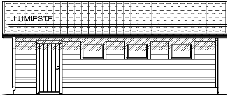
JULKISIVU 1.
